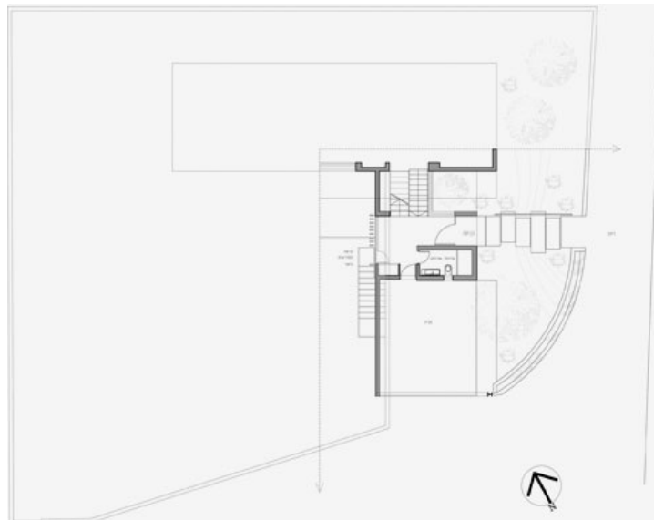
תוכנית מפלס הביניים, שאליו נכנסים מהרחוב ומקשר בין הקומות (שרטוט: יעקבס-יניב אדריכלים)
