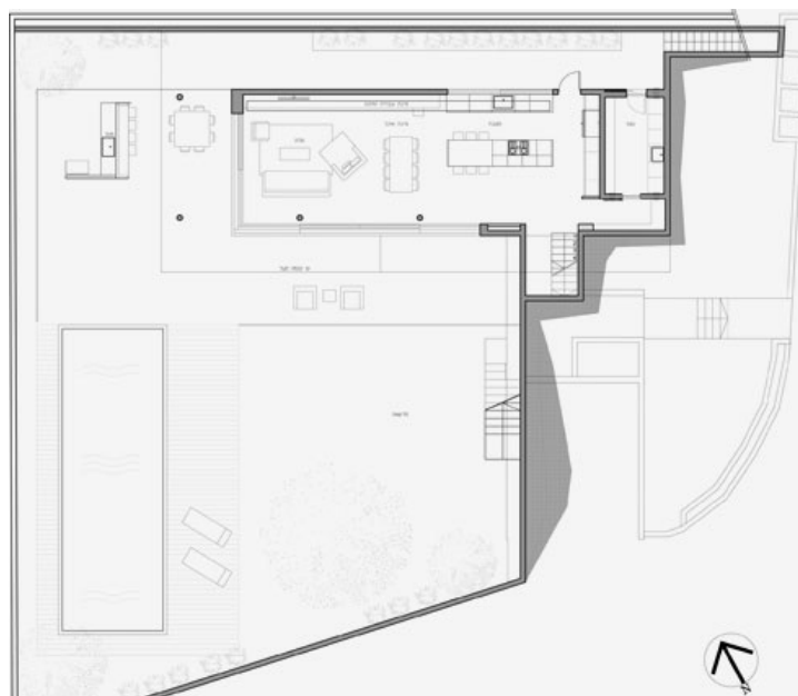
תוכנית הקומה התחתונה, שנמצאת במפלס הגינה והברכה (שרטוט: יעקבס-יניב אדריכלים)
