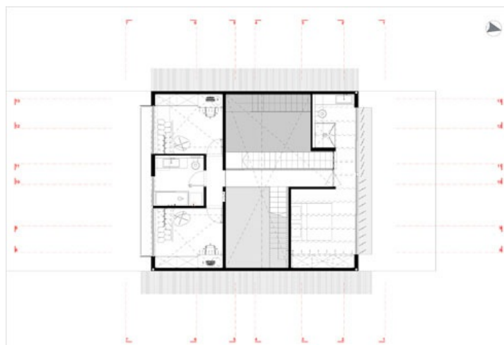
תוכנית הקומה הראשונה, שבה סוויטת ההורים והחלק התחתון של חדרי הבנות (תוכנית: ארכ' עדי וינברג - סטודיו ארביג'אז)
