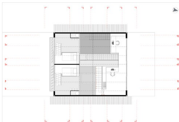
תוכנית קומת הגג, שבה גלריית השינה של הבנות ומשרד ביתי פתוח לחלל (תוכנית: ארכ' עדי וינברג - סטודיו ארביג'אז)
