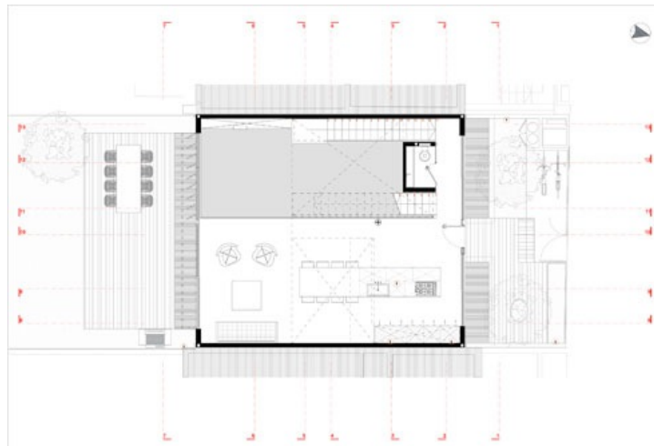
תוכנית קומת הכניסה, שבה המטבח (תוכנית: ארכ' עדי וינברג - סטודיו ארביג'אז)
